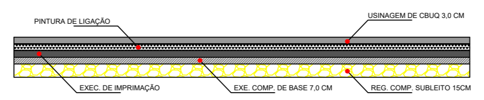
Seção Transversal - Avenida Escala s/s
