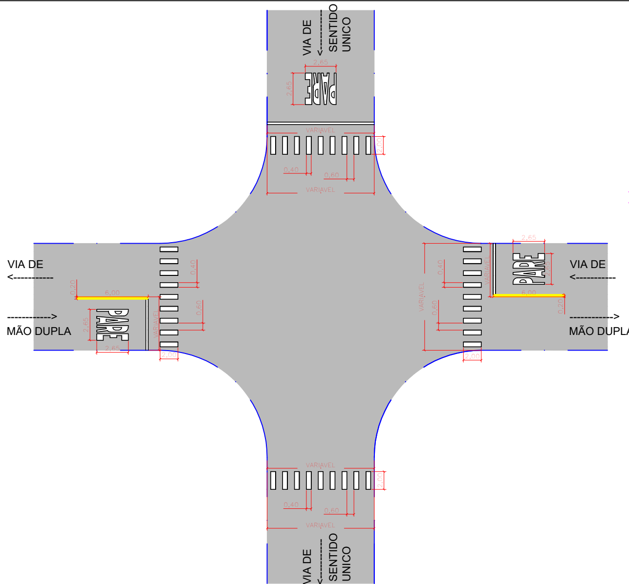
DETALHE SINALIZAÇÃO HORIZONTAL SEM ESCALA
