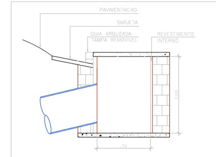
CORTE A-A POÇO DE VISITA SEM ESCALA
