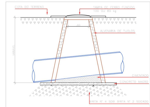
CORTE POÇO DE VISITA SEM ESCALA
